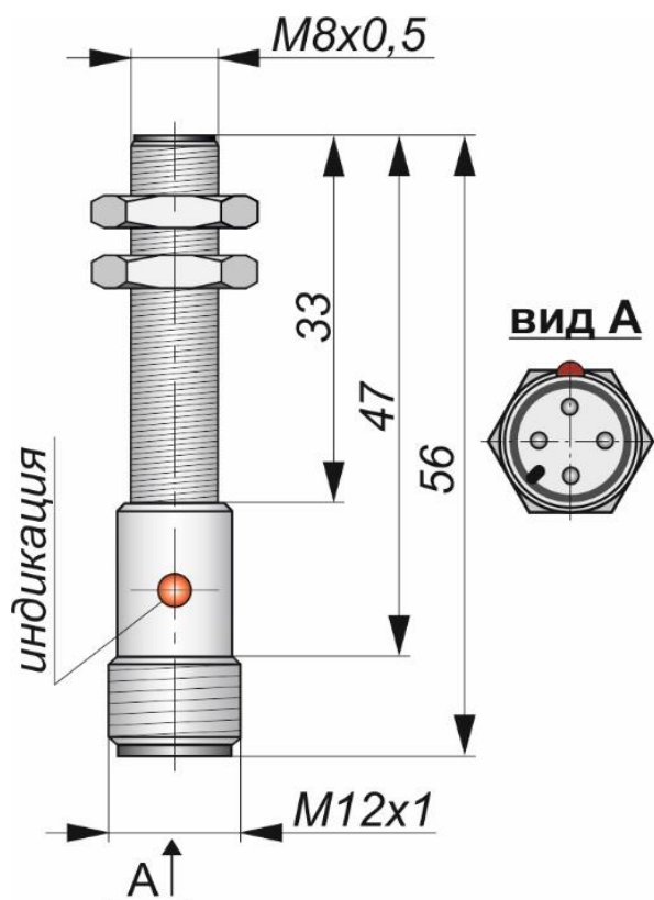
Габаритный чертеж
